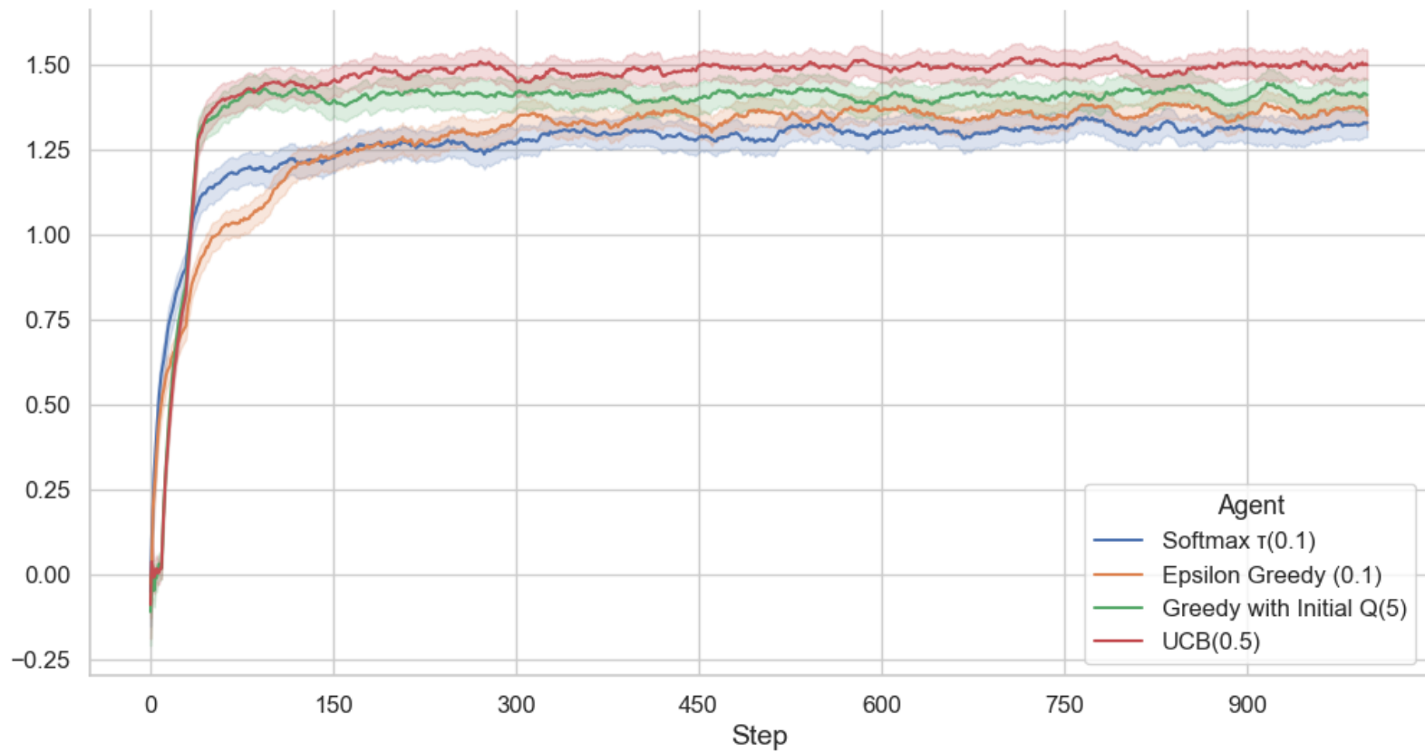
Best-tuned Parameters
